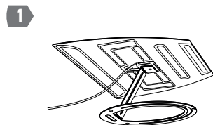
Установка антенны
